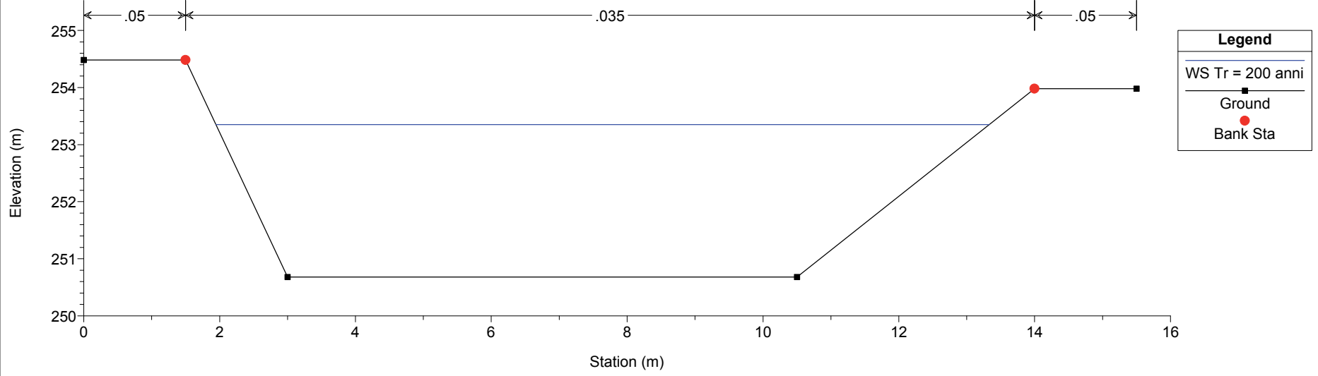
Cantogno Villafranca Plan: Plan 01 09/10/2017 River = T. Cantogno Reach = Villafranca RS = 12 Sezione 12 Can
