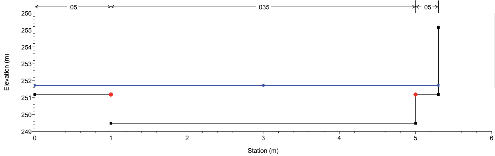
Canale del Martinetto Plan: Plan 05 16/04/2018 River = Canale del Marti Reach = Villafranca P. RS = 9 Sezione 8 Ma a monte del 2° canale coperto
