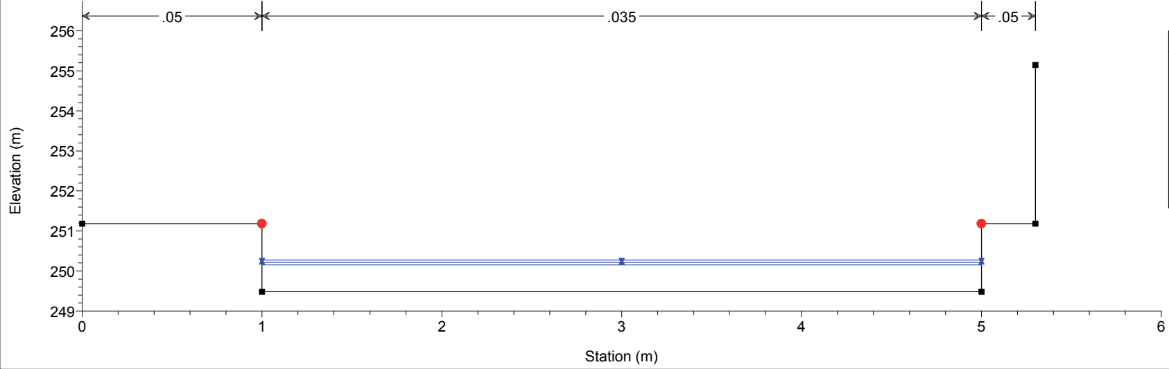
Canale del Martinetto Plan: Plan 04 06/10/2017 River = Canale del Marti Reach = Villafranca P. RS = 9 Sezione 8 Ma a monte del 2° canale coperto
