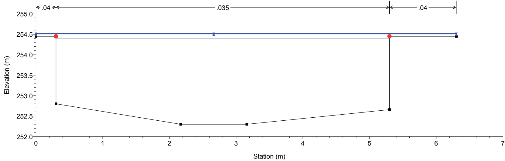
Bealera del Molino Villafranca P. Plan: Plan 07 13/04/2018 River = Bealera del Moli Reach = Villafranca Piem RS = 20 sezione 9B Mo valle ponte scuole
