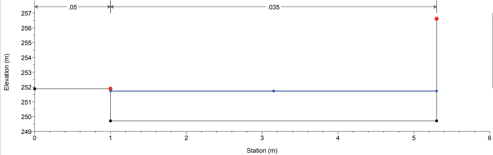
Canale del Martinetto Plan: Plan 05 16/04/2018 River = Canale del Marti Reach = Villafranca P. RS = 11 Sezione a valle del ponte 6B Ma
