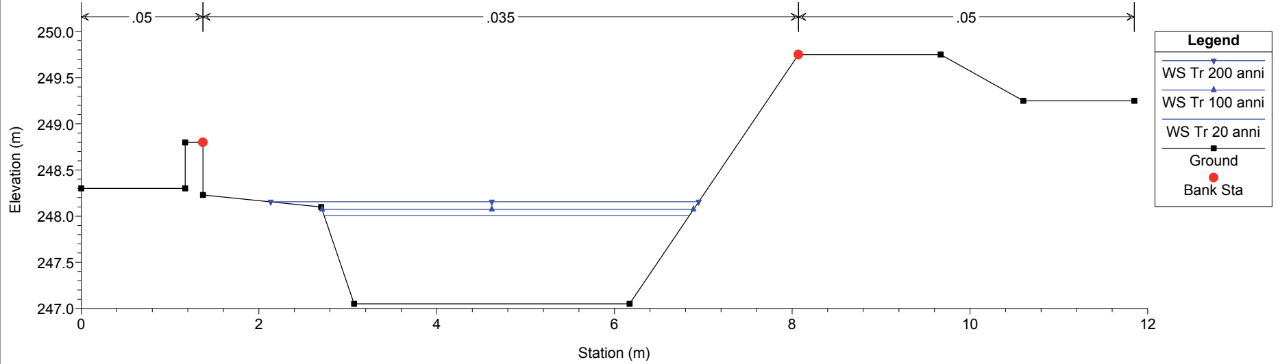
Canale del Martinetto Plan: Plan 04 06/10/2017 River = Canale del Marti Reach = Villafranca P. RS = 3 Sezione 12 Ma
