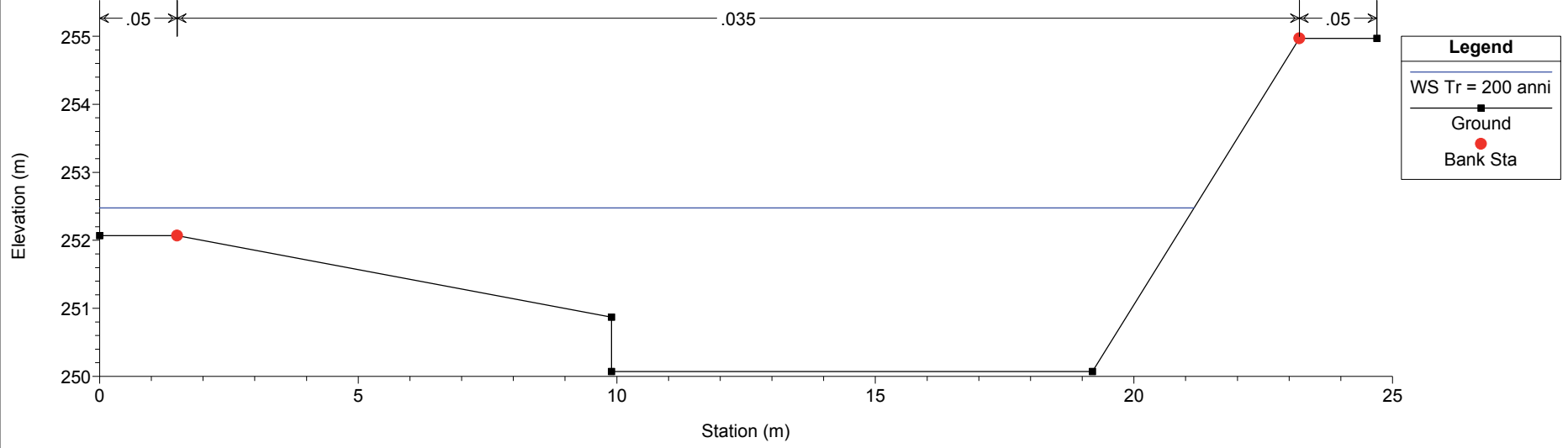
Cantogno Villafranca Plan: Plan 01 09/10/2017 River = T. Cantogno Reach = Villafranca RS = 8 Sezione 8 Can
