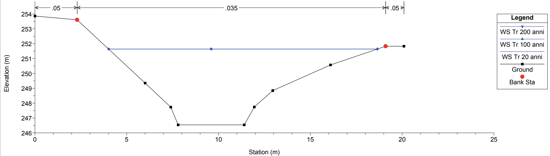
Canale del Martinetto Plan: Plan 05 16/04/2018 River = Canale del Marti Reach = Villafranca P. RS = 3 Sezione 12 Ma
