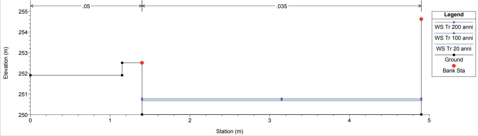
Canale del Martinetto Plan: Plan 04 06/10/2017 River = Canale del Marti Reach = Villafranca P. RS = 13 Sezione 5 Ma
