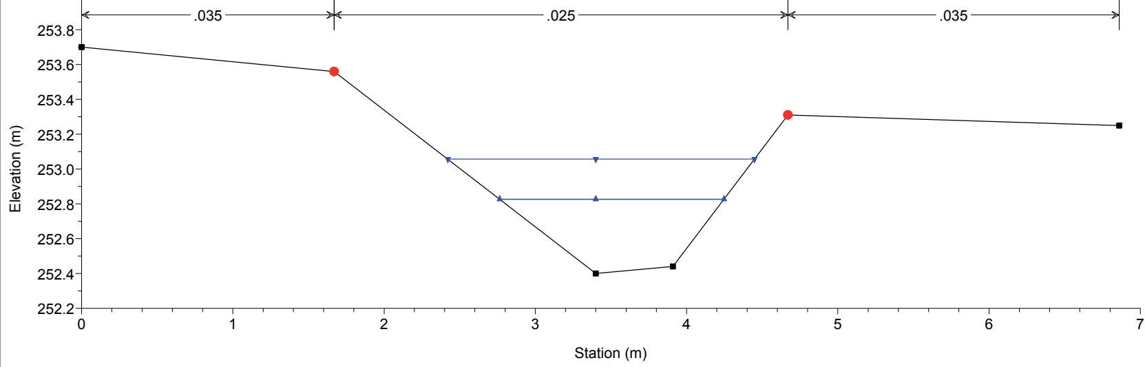
Canale Via Carando Plan: Plan 04 06/04/2018 River = Canale Via Caran Reach = Villafranca P. RS = 9 Sezione n. 4 Ca
