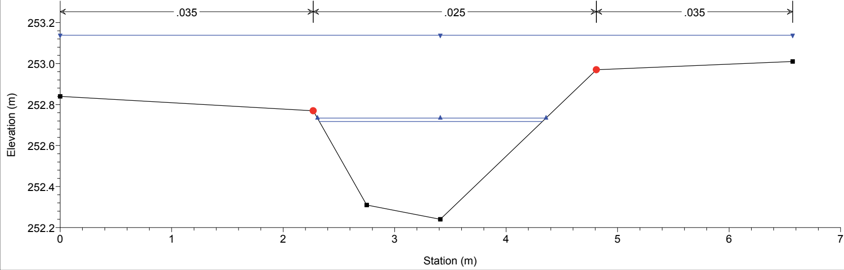
Canale Via Carando Plan: Plan 05 16/04/2018 River = Canale Via Caran Reach = Villafranca P. RS = 9 Sezione n. 4 Ca
