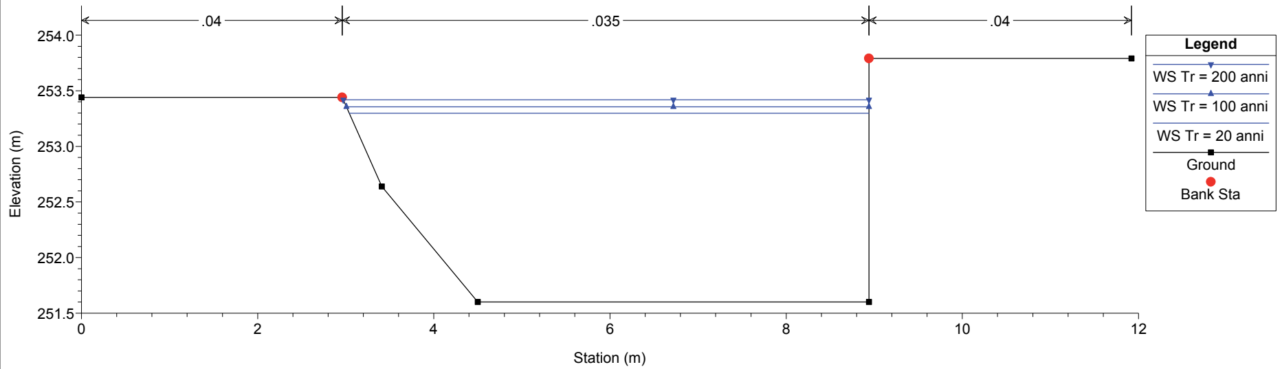
Bealera del Molino Villafranca P. Plan: Plan 08 16/04/2018 River = Bealera del Moli Reach = Villafranca Piem RS = 13.5 Sezione 14bis Mo
