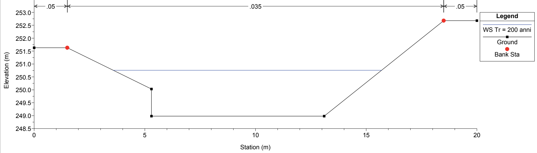
Cantogno Villafranca Plan: Plan 01 09/10/2017 River = T. Cantogno Reach = Villafranca RS = 2 Sezione 2 Can
