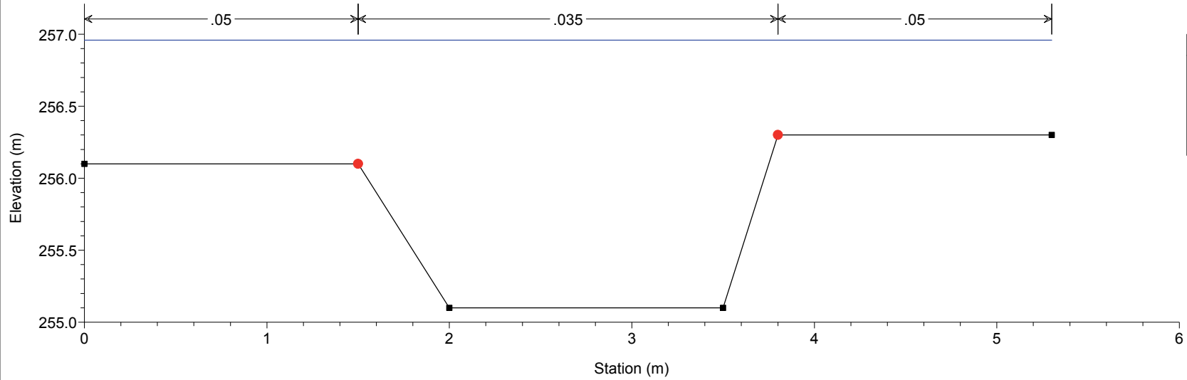
Sterpissone Villafranca Plan: Plan 01 10/10/2017 River = T.Sterpissone Reach = Villafranca RS = 9 Sezione 9 Ste
