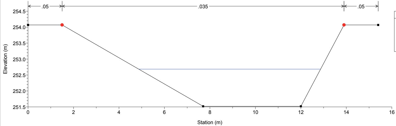
Sterpissone Villafranca Plan: Plan 01 10/10/2017 River = T.Sterpissone Reach = Villafranca RS = 5 Sezione 5 Ste
