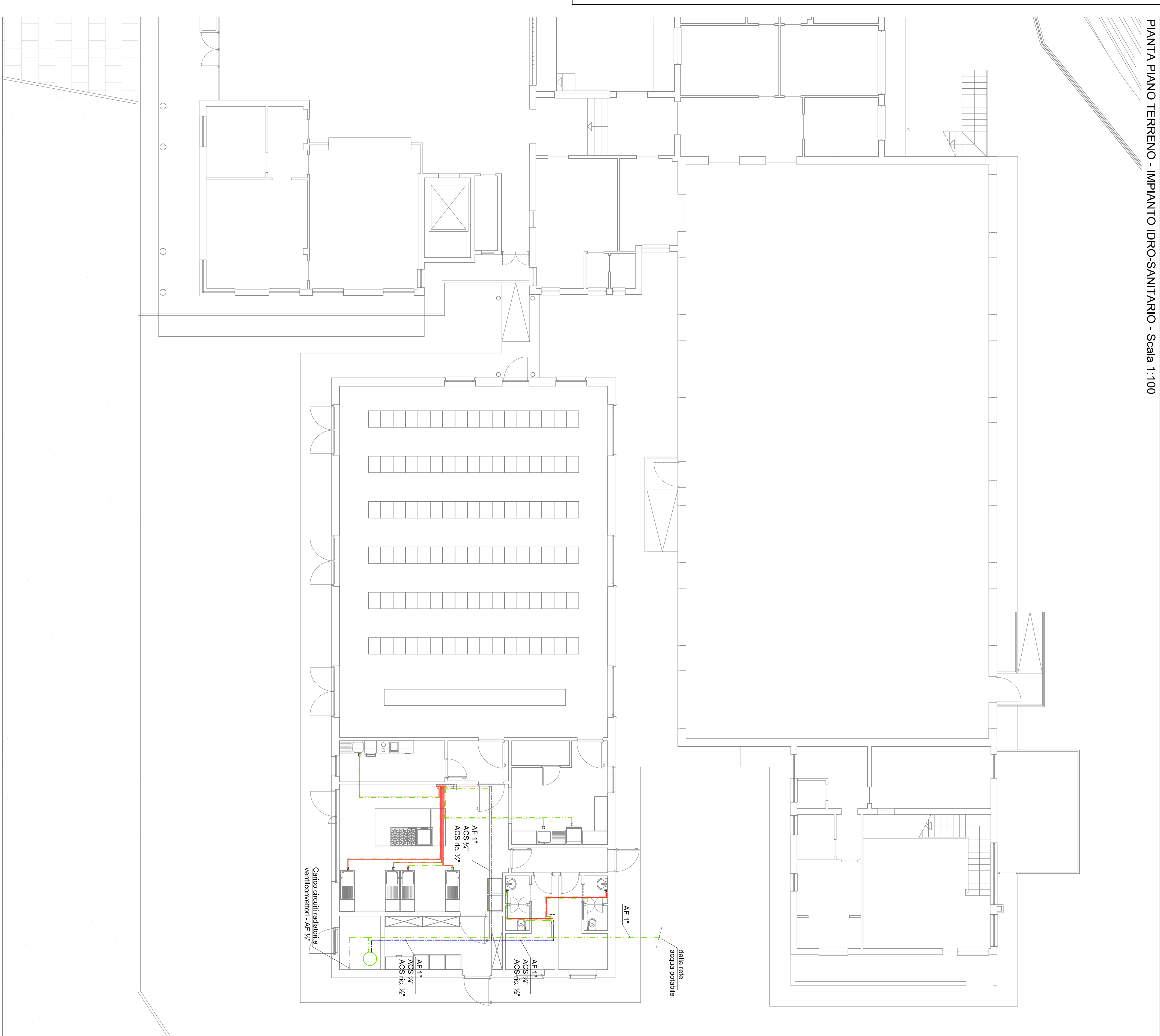
PIANTA PIANO TERRENO - IMPIANTO SCARICHI - Scala 1:100
