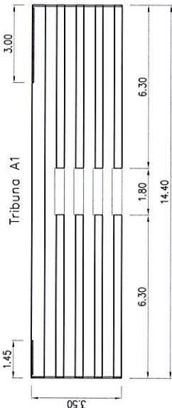
Piante scala 1:100
